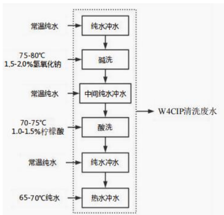
图 2-5 CIP 清洗工艺流程
