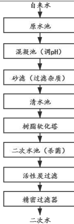
图 2-1 纯水制备工艺流程图
