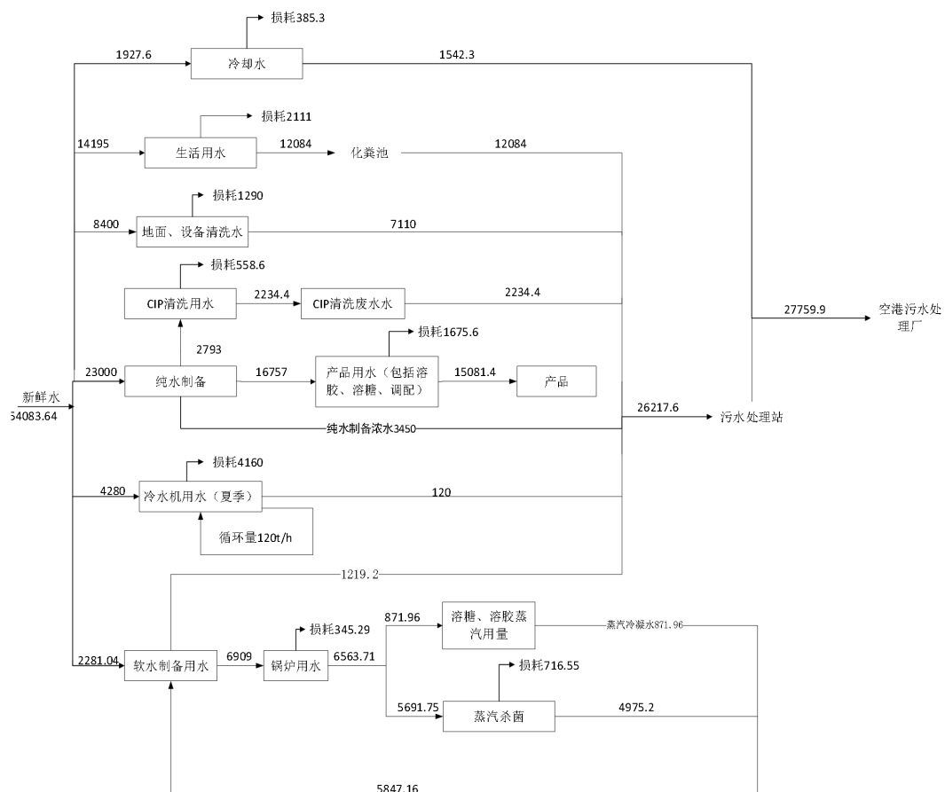
图 2-3 本项目建成后全厂水平衡图 (t/a)
