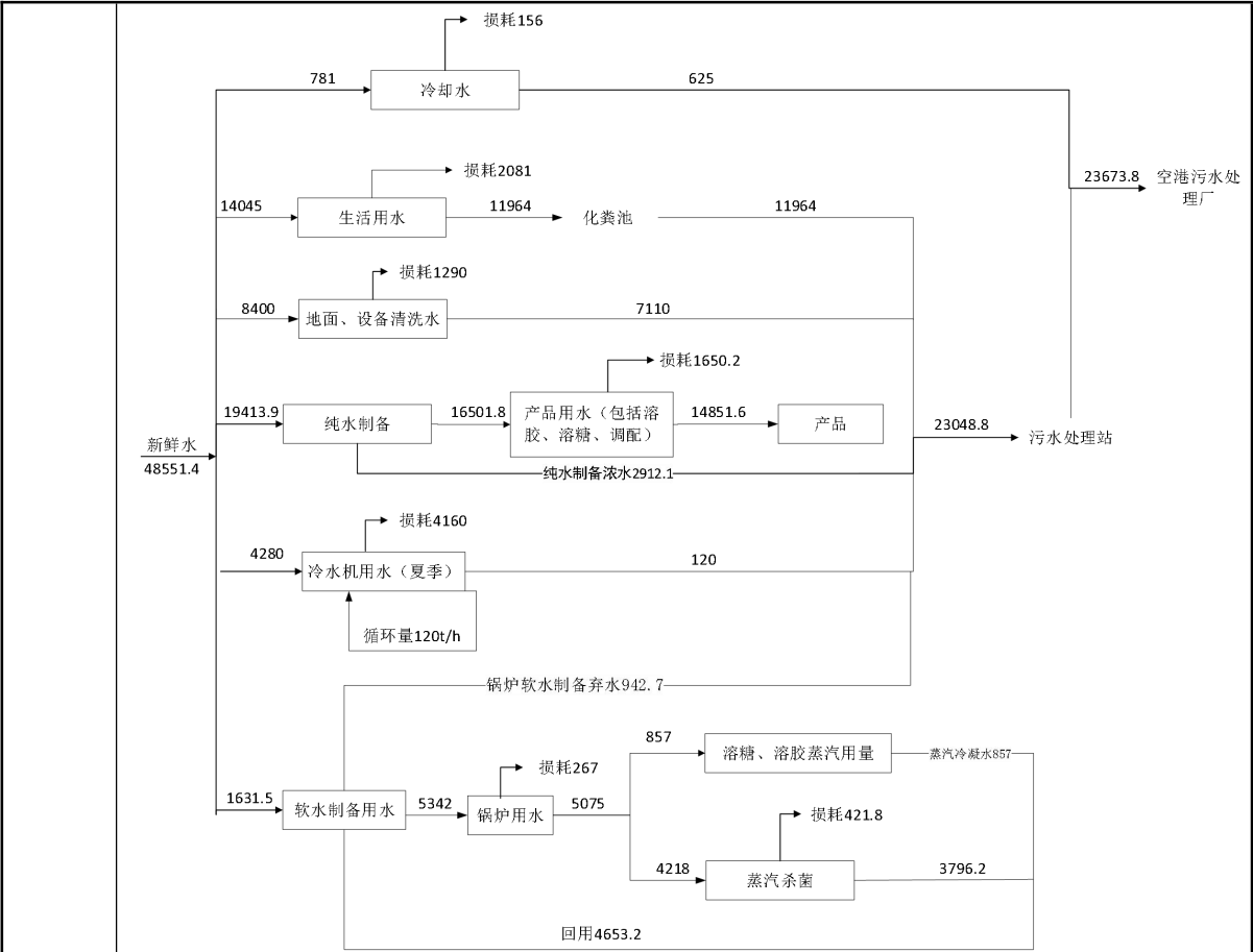
图 2-8 现有项目水平衡图
