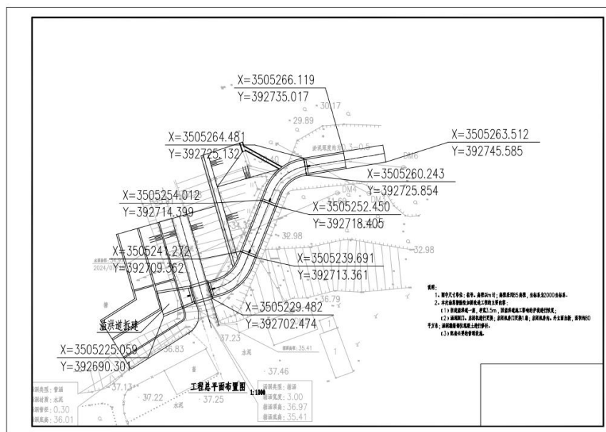
图 1-5 油菜塘工程平面布置图（含拐点坐标）
